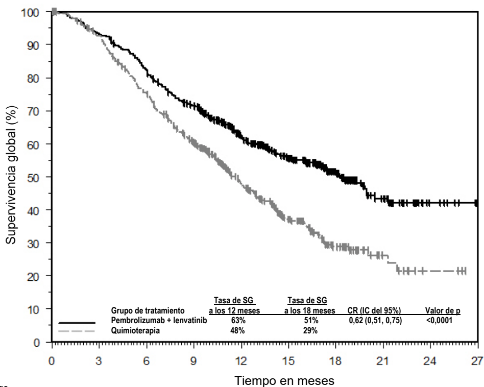
Figura 32: Curva de Kaplan-Meier para la supervivencia global por grupo de tratamiento en el ensayo KEYNOTE-775 (población con intención de tratar)
