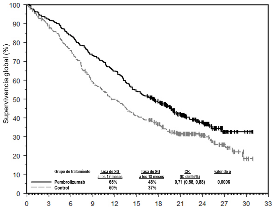
Figura 11: Curva de Kaplan-Meier para la supervivencia global en el ensayo KEYNOTE-407
