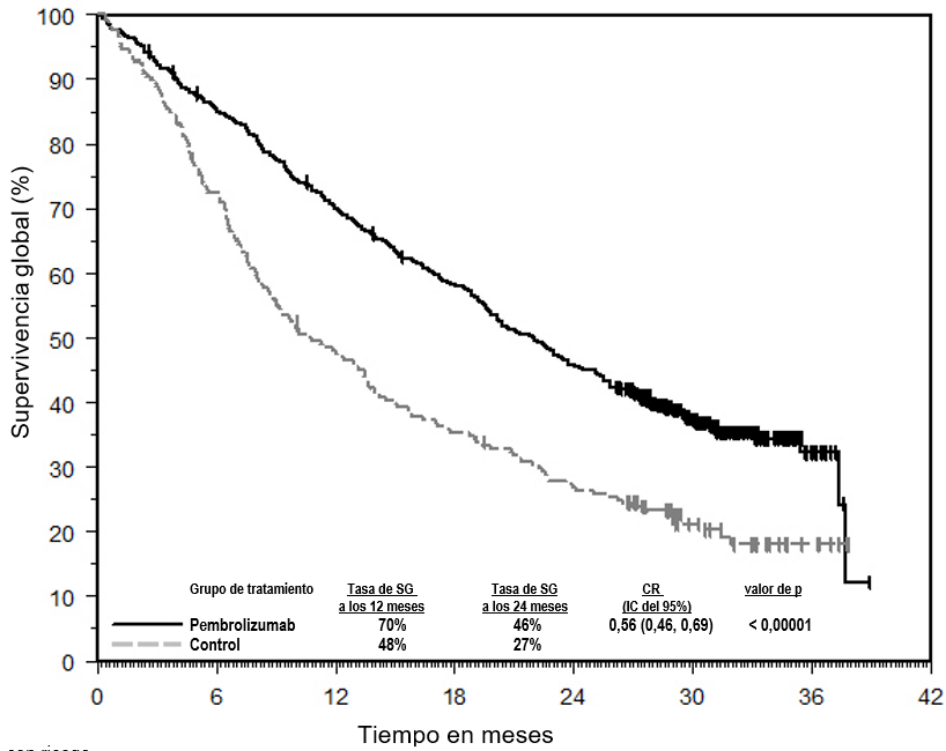
Figura 9: Curva de Kaplan-Meier para la supervivencia global por grupo de tratamiento en el ensayo KEYNOTE-189 (población con intención de tratar)
