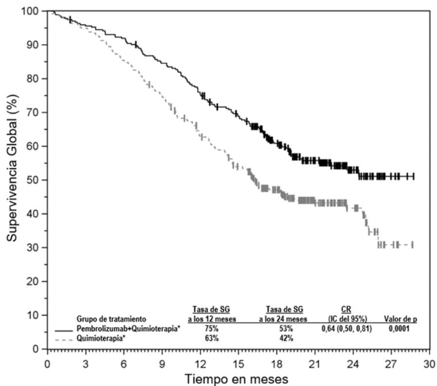
Figura 34: Curva de Kaplan-Meier para la supervivencia global por grupo de tratamiento en el ensayo KEYNOTE-826 para pacientes con expresión PD-L1 (CPS \geq 1)
