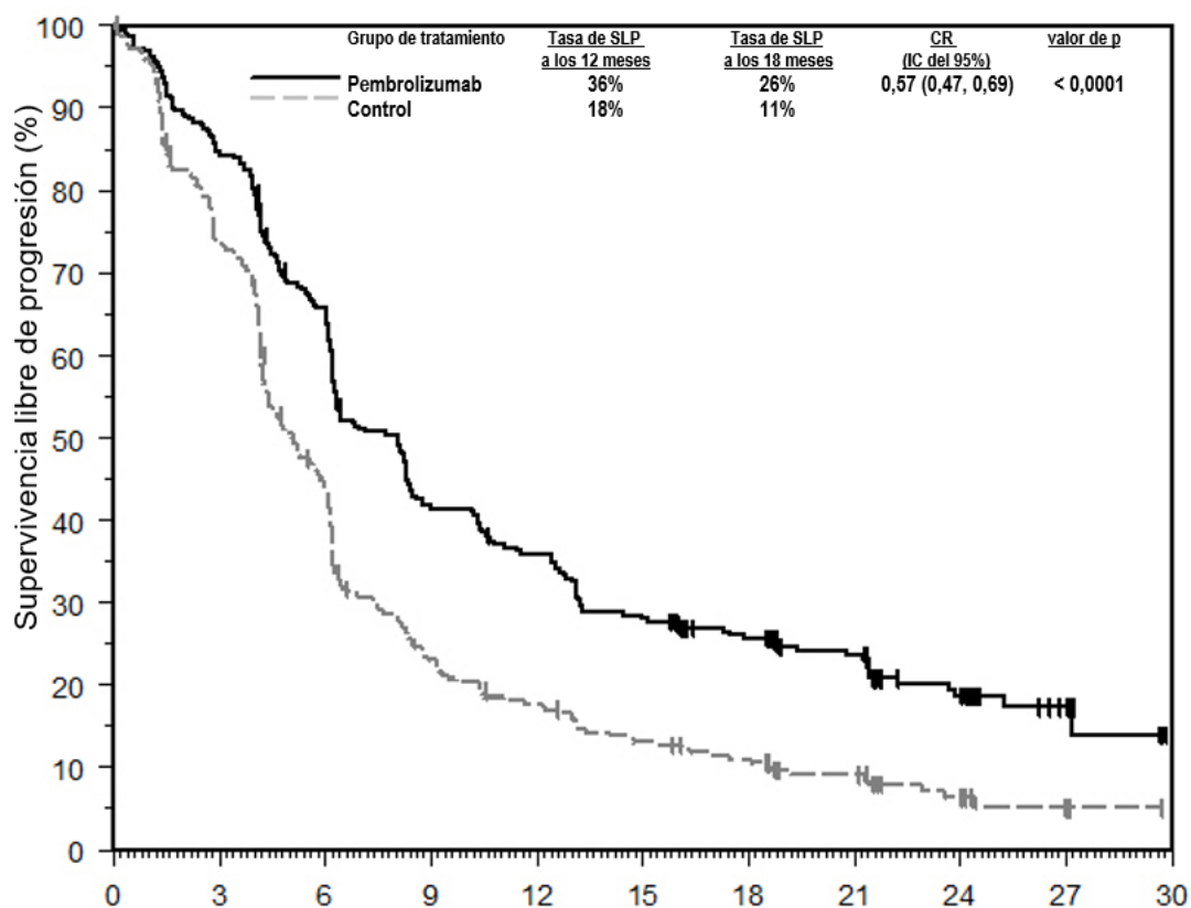
Figura 12: Curva de Kaplan-Meier para la supervivencia libre de progresión en el ensayo KEYNOTE-407
