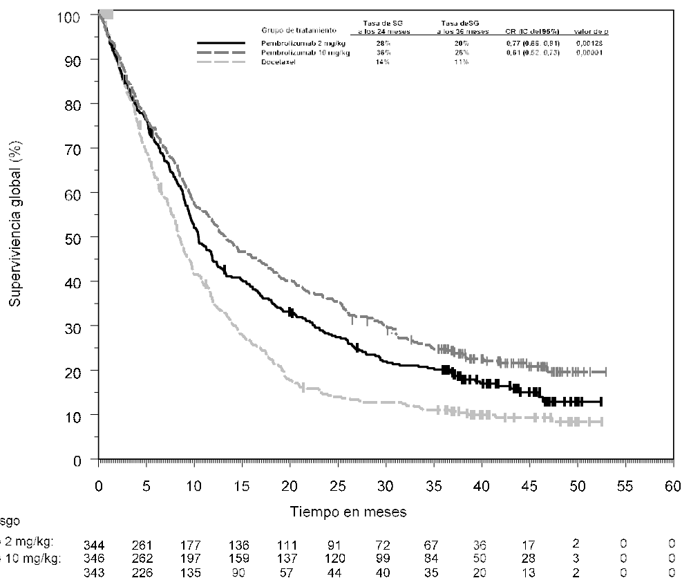
Figura 13: Curva de Kaplan-Meier para la supervivencia global por grupo de tratamiento en el ensayo KEYNOTE-010 (pacientes con TPS ≥ 1% de expresión de PD-L1, población con intención de tratar)
