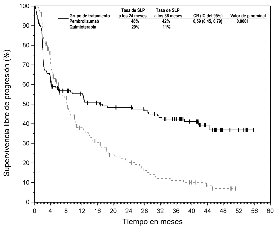
Figura 26: Curva de Kaplan-Meier para la supervivencia libre de progresión por grupo de tratamiento en el ensayo KEYNOTE-177 (población con intención de tratar)
