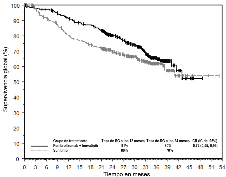
Figura 24: Curva de Kaplan-Meier para la supervivencia global por grupo de tratamiento en el ensayo KEYNOTE-581
