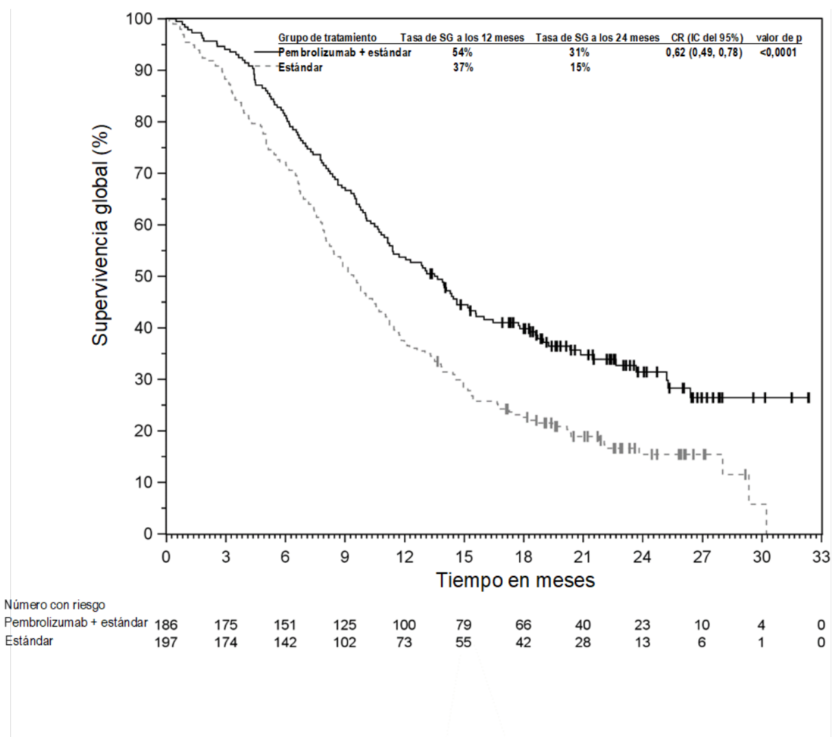
Figura 28: Curva de Kaplan-Meier para la supervivencia global por grupo de tratamiento en pacientes del ensayo KEYNOTE-590 con expresión de PD-L1 (CPS \geq 10)
