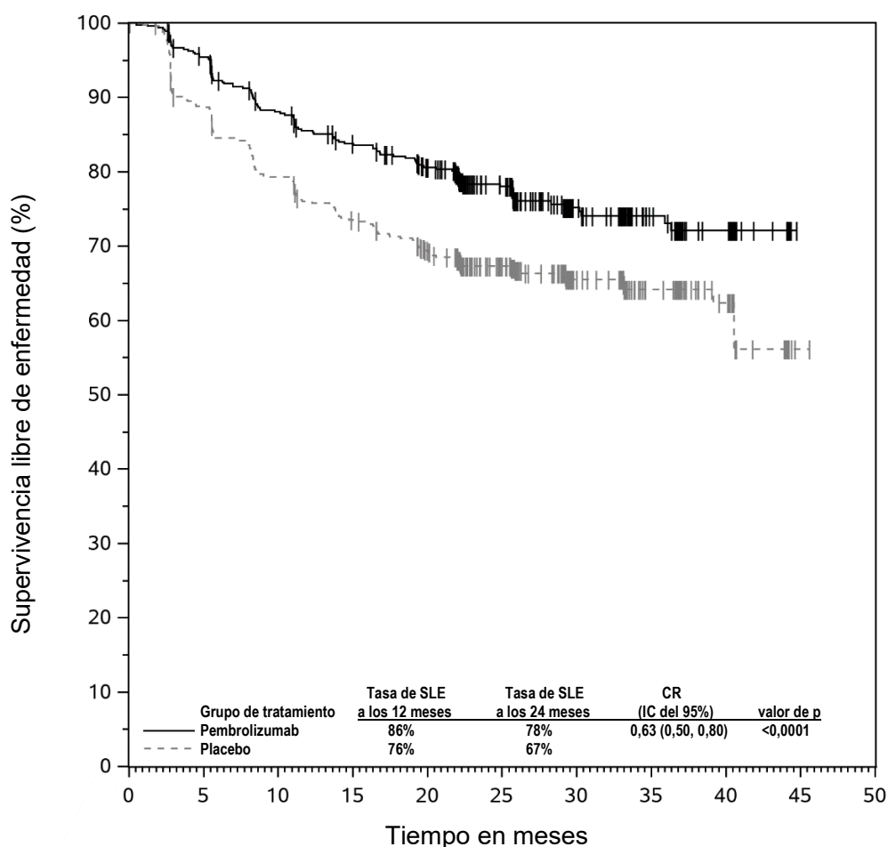
Figura 25: Curva de Kaplan-Meier para la supervivencia libre de enfermedad por grupo de tratamiento en el ensayo KEYNOTE-564 (población con intención de tratar)*
