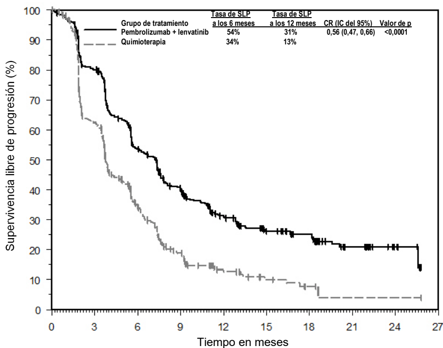
Figura 33: Curva de Kaplan-Meier para la supervivencia libre de progresión por grupo de tratamiento en el ensayo KEYNOTE-775 (población con intención de tratar)
