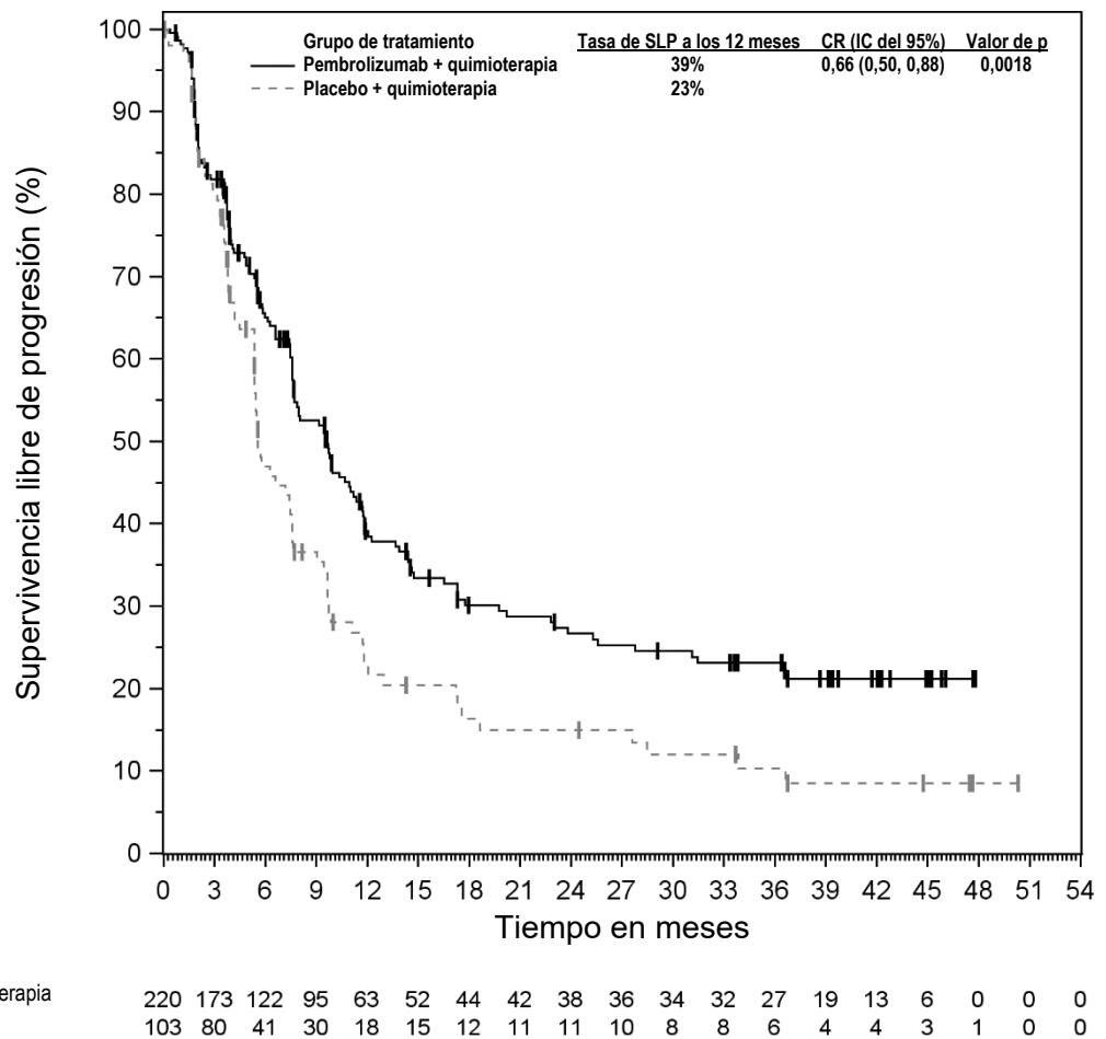
Figura 30: Curva de Kaplan-Meier para la supervivencia libre de progresión por grupo de tratamiento en pacientes del ensayo KEYNOTE-355 con expresión de PD-L1 (CPS \geq 10)
