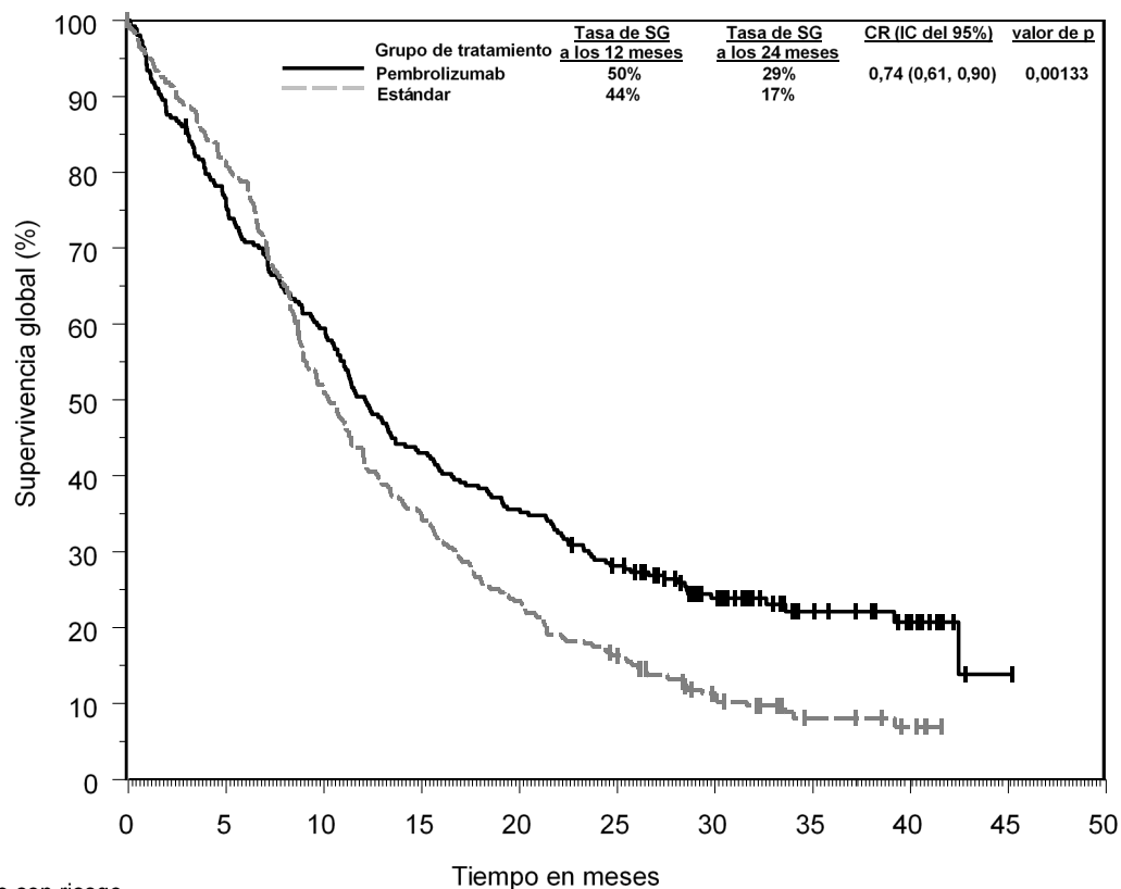
Figura 19: Curva de Kaplan-Meier para la supervivencia global de pembrolizumab en monoterapia en pacientes del ensayo KEYNOTE-048 con expresión de PD-L1 (CPS \geq 1)
