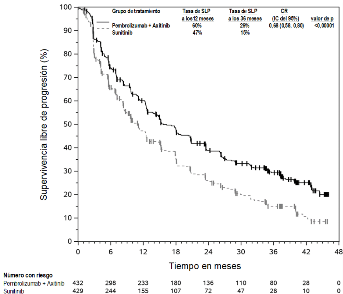
Figura 22: Curva de Kaplan-Meier para la supervivencia libre de progresión por grupo de tratamiento en el ensayo KEYNOTE-426 (población con intención de tratar)
