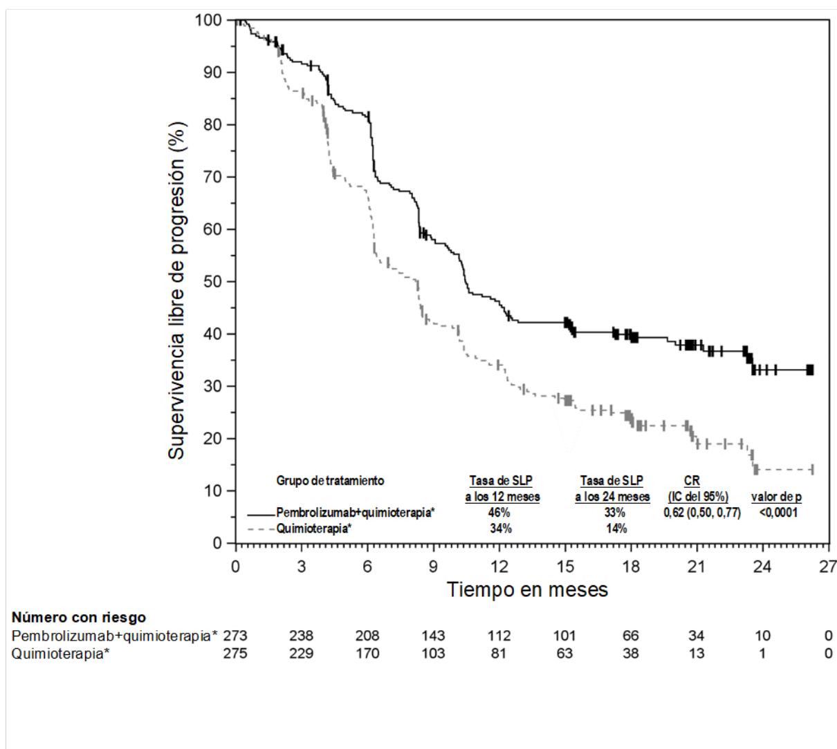
Figura 35: Curva de Kaplan-Meier para la supervivencia libre de progresión por grupo de tratamiento en el ensayo KEYNOTE-826 para pacientes con expresión PD-L1 (CPS \geq 1)
