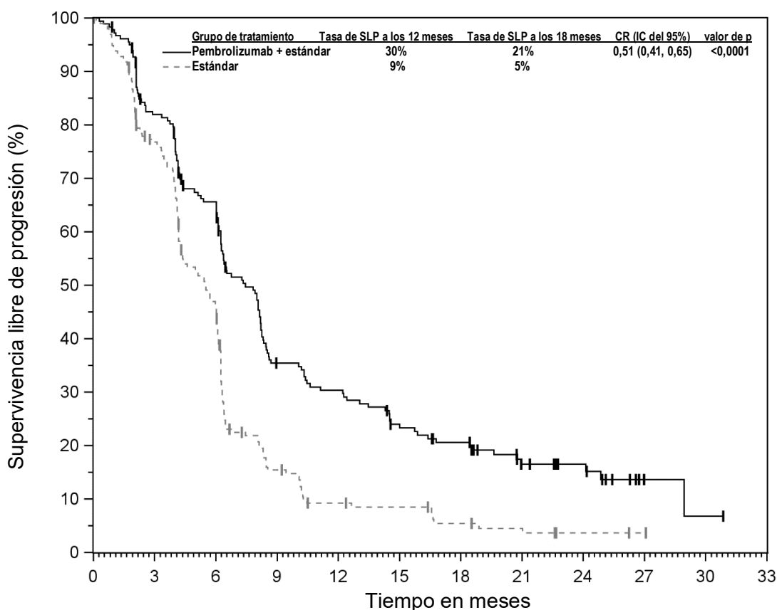
Figura 29: Curva de Kaplan-Meier para la supervivencia libre de progresión por grupo de tratamiento en pacientes del ensayo KEYNOTE-590 con expresión de PD-L1 (CPS ≥ 10)
