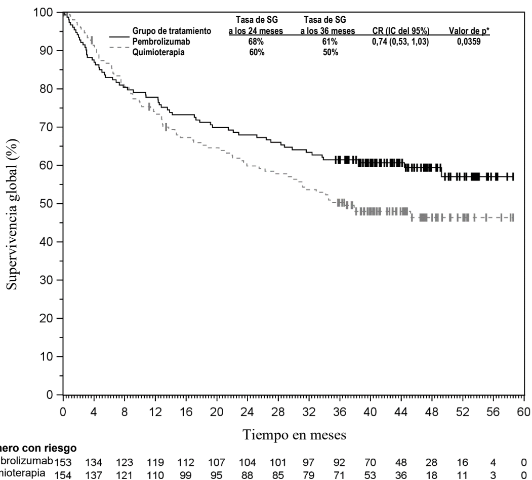
Figura 27: Curva de Kaplan-Meier para la supervivencia global por grupo de tratamiento en el ensayo KEYNOTE-177 (población con intención de tratar)
