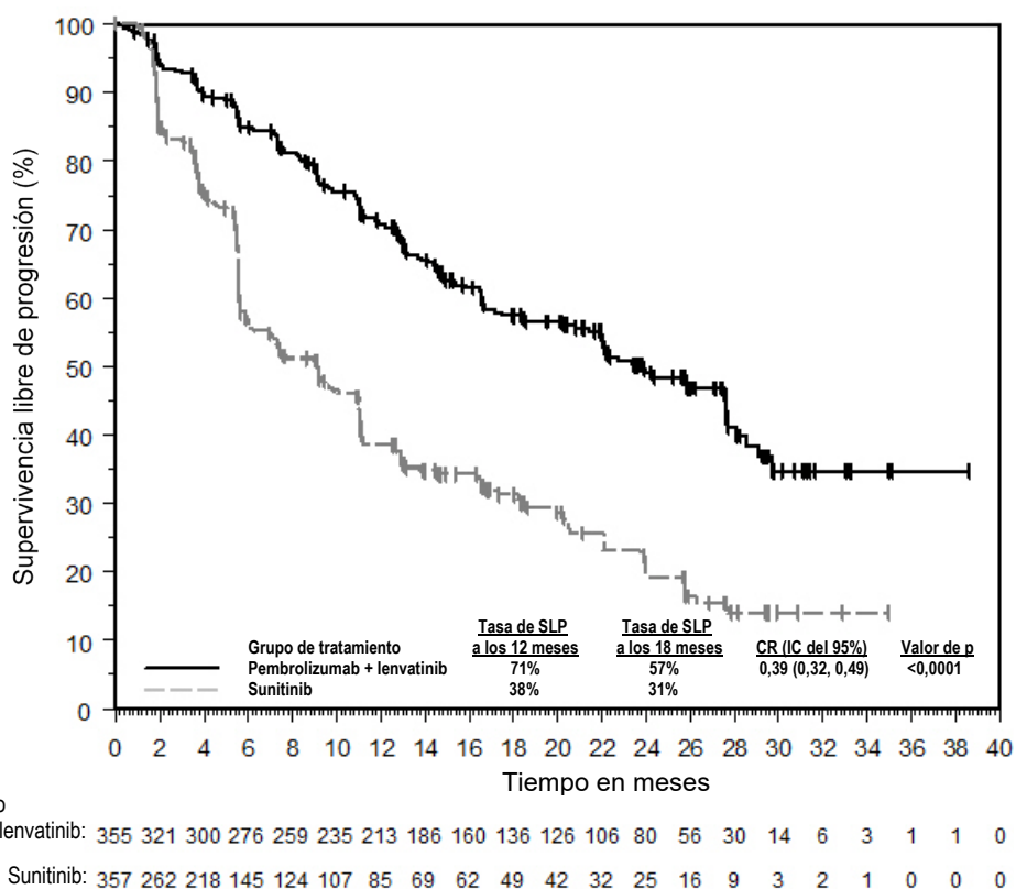
Figura 23: Curva de Kaplan-Meier para la supervivencia libre de progresión por grupo de tratamiento en el ensayo KEYNOTE-581
