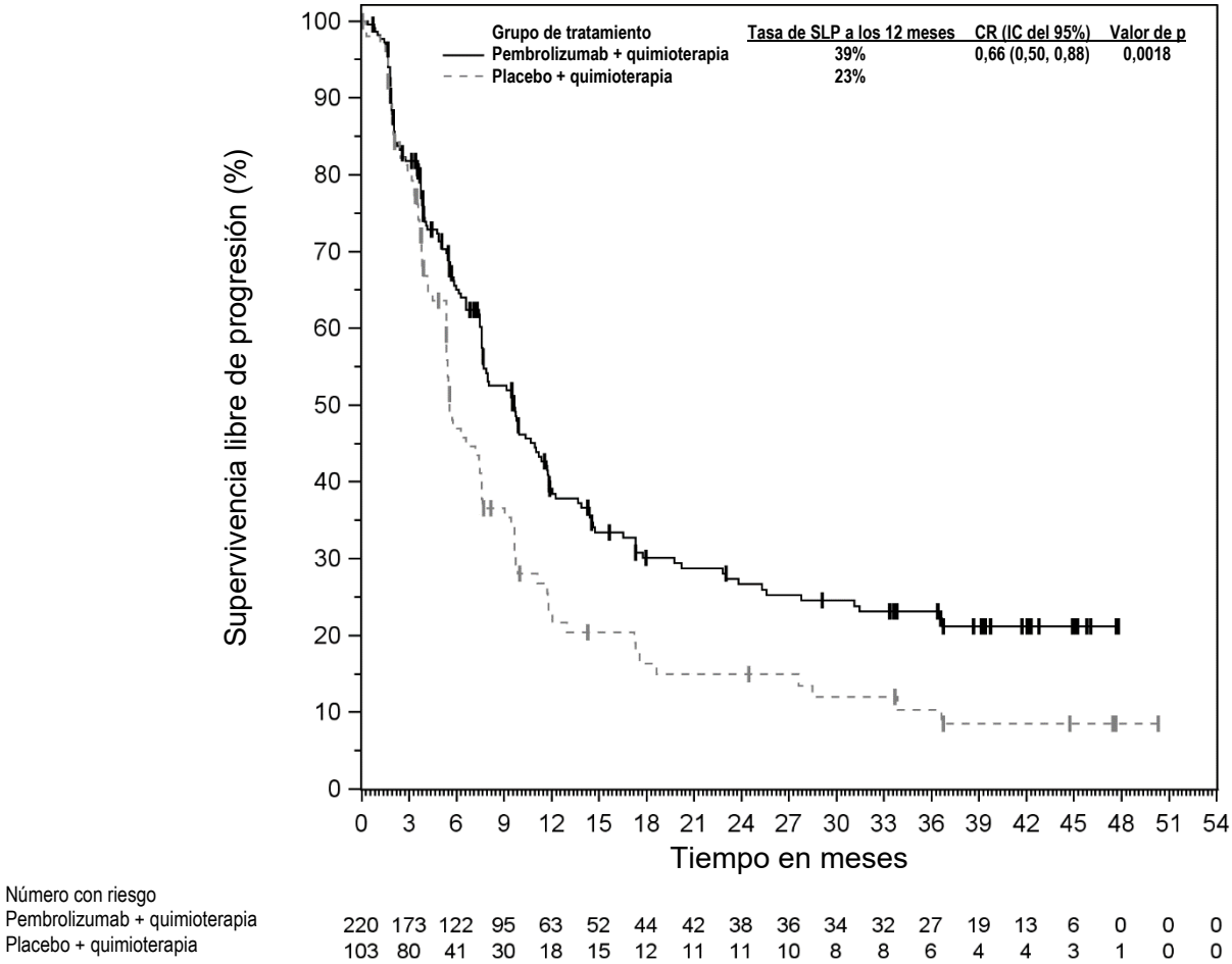
Figura 40. Curva de Kaplan-Meier para la supervivencia libre de progresión por grupo de tratamiento en pacientes del ensayo KEYNOTE-355 con expresión de PD-L1 (CPS ≥ 10)
