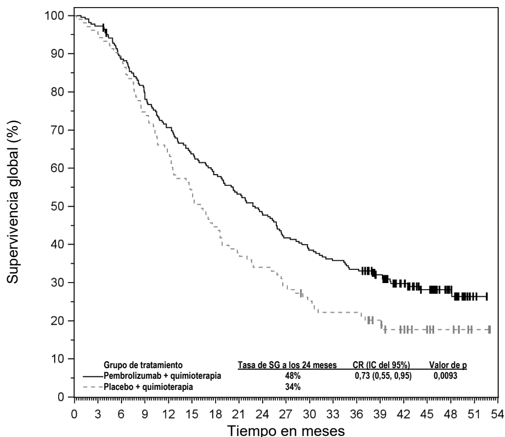
Figura 41. Curva de Kaplan-Meier para la supervivencia global por grupo de tratamiento en pacientes del ensayo KEYNOTE-355 con expresión de PD-L1 (CPS \geq 10 )
